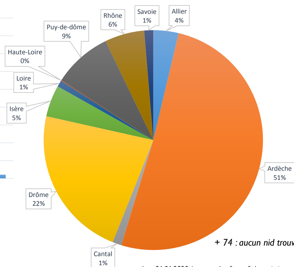
Proportion du nombre de nids trouvés en RA par département en 2019
