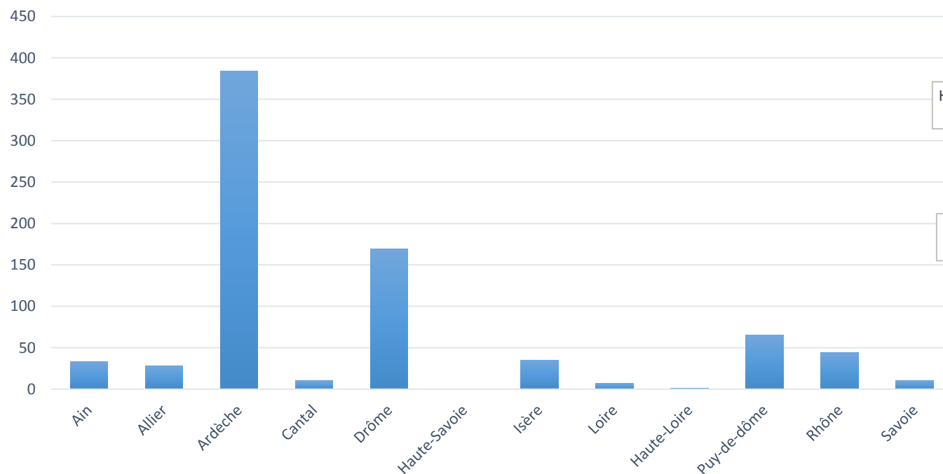
Nombre de nids découverts par département sur 2019
