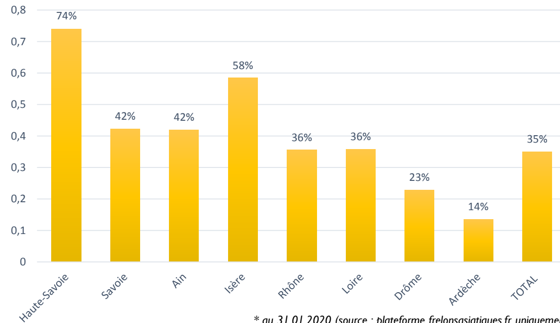
Taux d'erreur de signalement par département en 2019
