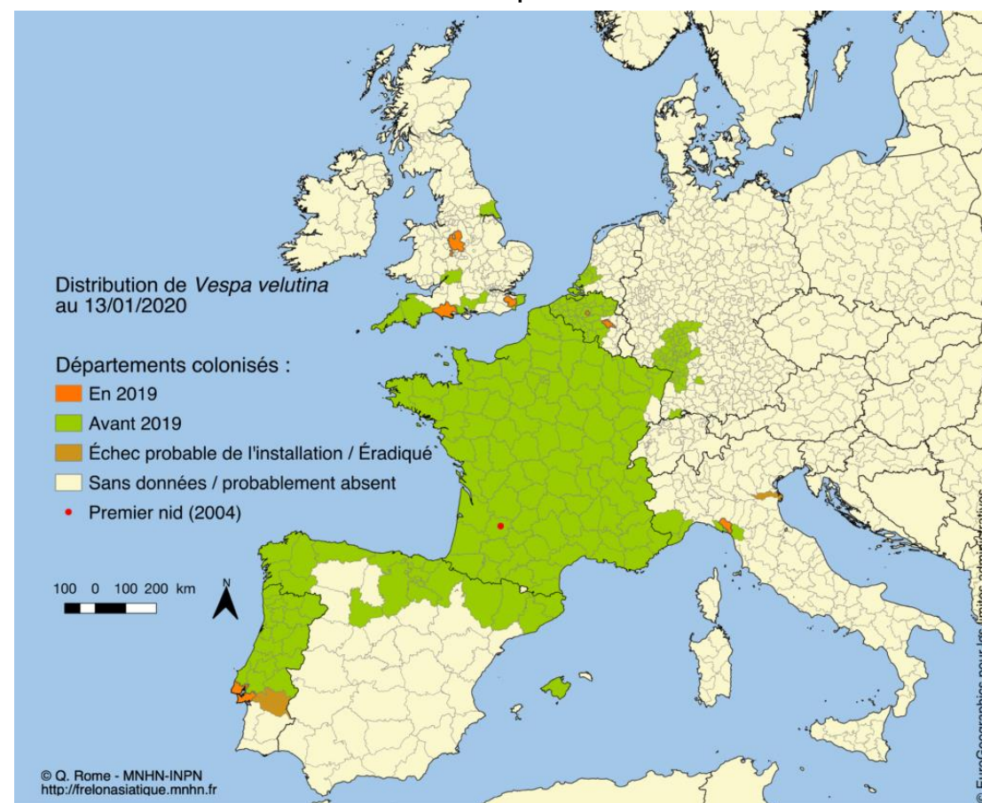
Distribution du Frelon asiatique en France au 13/01/20
